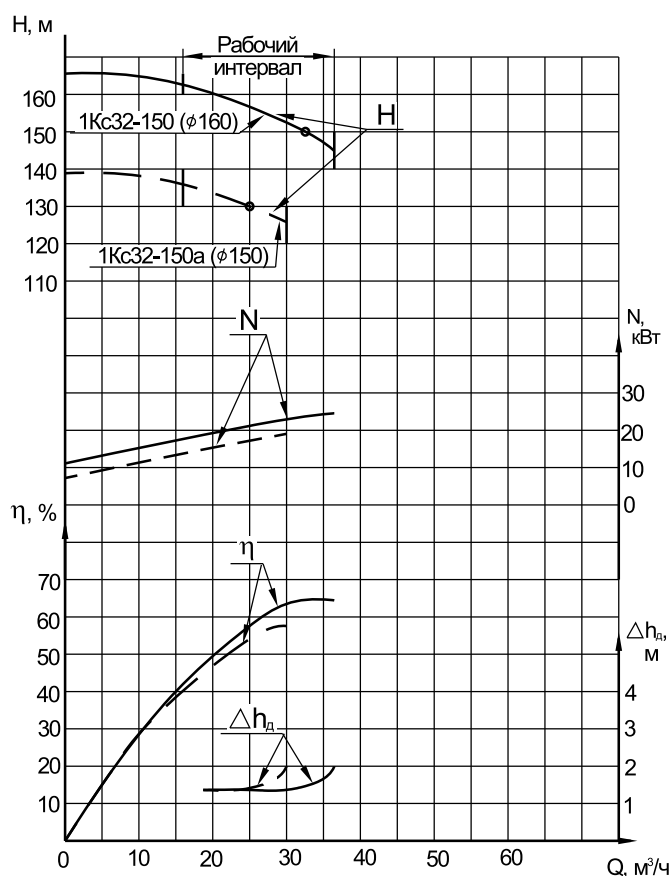
ХАРАКТЕРИСТИКА НАСОСА 1Kc32-150
