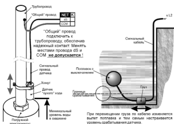
Варианты использования датчиков "сухого" хода
