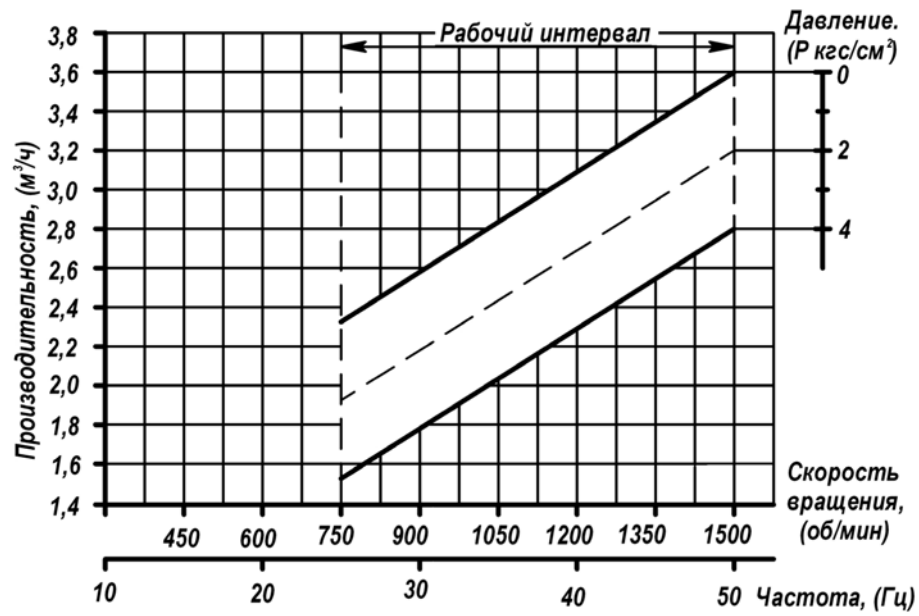
Электронасос Бурун СХ 3,6/4- Ч (ЧМ) 0,75/4
