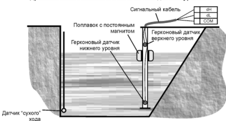
Дренаж с использованием поплавкового датчика уровня
