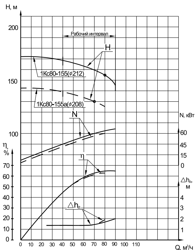
ХАРАКТЕРИСТИКА НАСОСА 1Kc80-155
