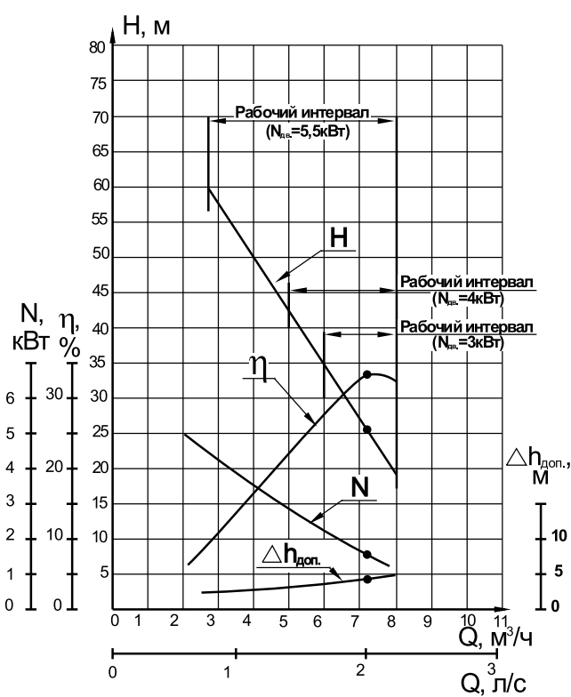
БК2/26, ВКС2/26, ВКО2/26 частота вращения — 24 с -1 (1450 об/мин)
