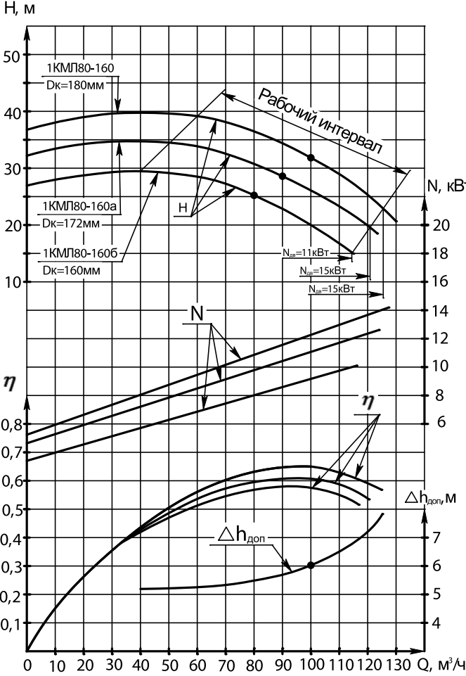
Характеристика электронасоса 1КМЛ80-160 на воде t=293K (20°C), ρ=1000кг/м³, n=48,3 с⁻¹(2900 об/мин)
