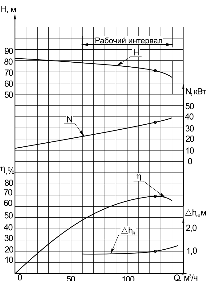
ХАРАКТЕРИСТИКА АГРЕГАТОВ 1КсВ 125-71-1
