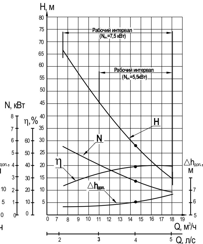
БК4/28, ВКС4/28, ВКО4/28 частота вращения — 24 с -1 (1450 об/мин)
