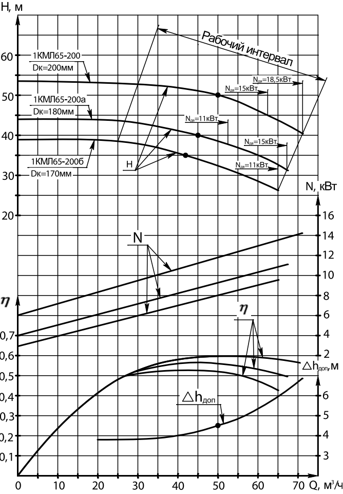
Характеристика насоса 1КМЛ65-200 на воде t=293K (20°C), ρ=1000кг/м³, n=48,3 с⁻¹(2900 об/мин)
