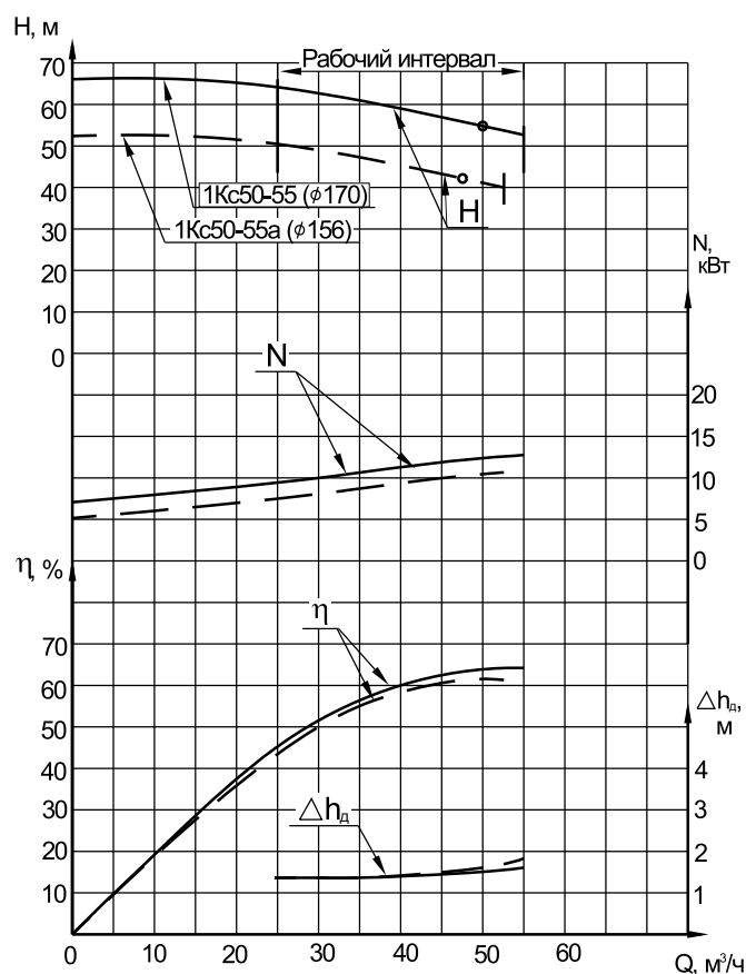
ХАРАКТЕРИСТИКА НАСОСА 1Kc50-55
