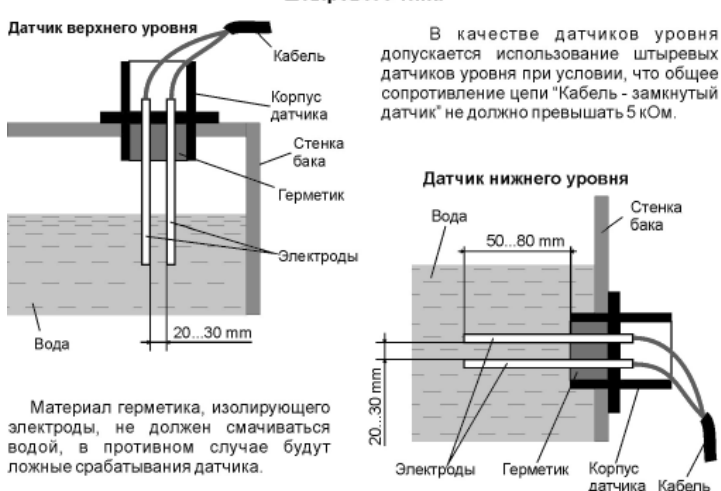
Дренаж с использованием штыревых датчиков уровня
