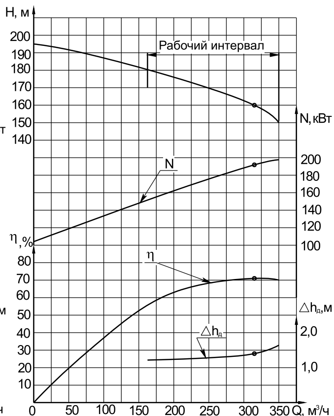
ХАРАКТЕРИСТИКА АГРЕГАТОВ 1КсВ 315-160-1
