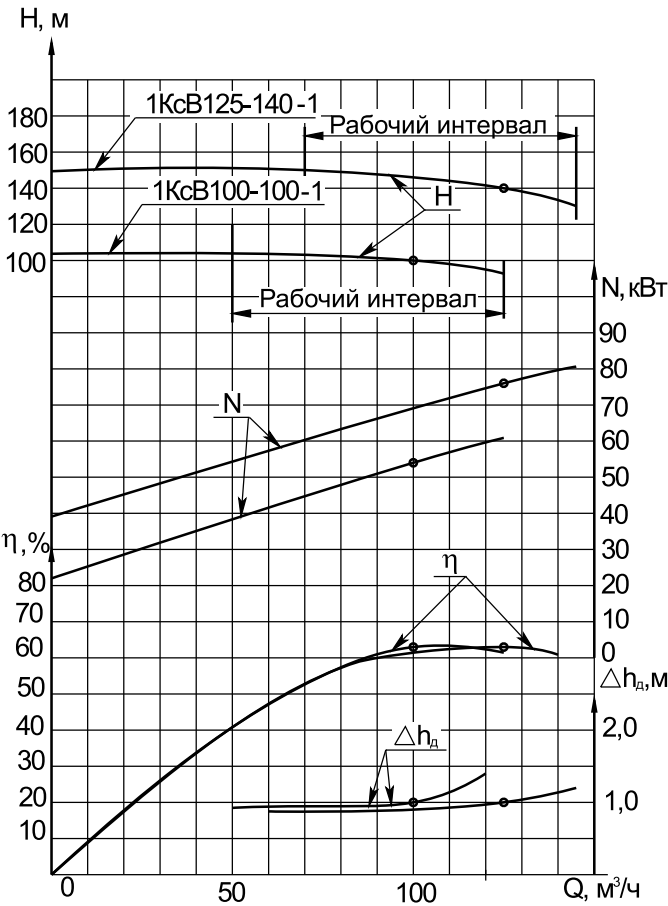
ХАРАКТЕРИСТИКА АГРЕГАТОВ 1КсВ 125-140-1 и 1КсВ 100-100-1
