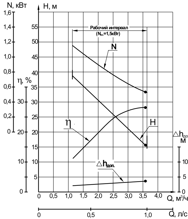
БК1/16, ВКС1/16, ВКО1/16 частота вращения — 24 с -1 (1450 об/мин)
