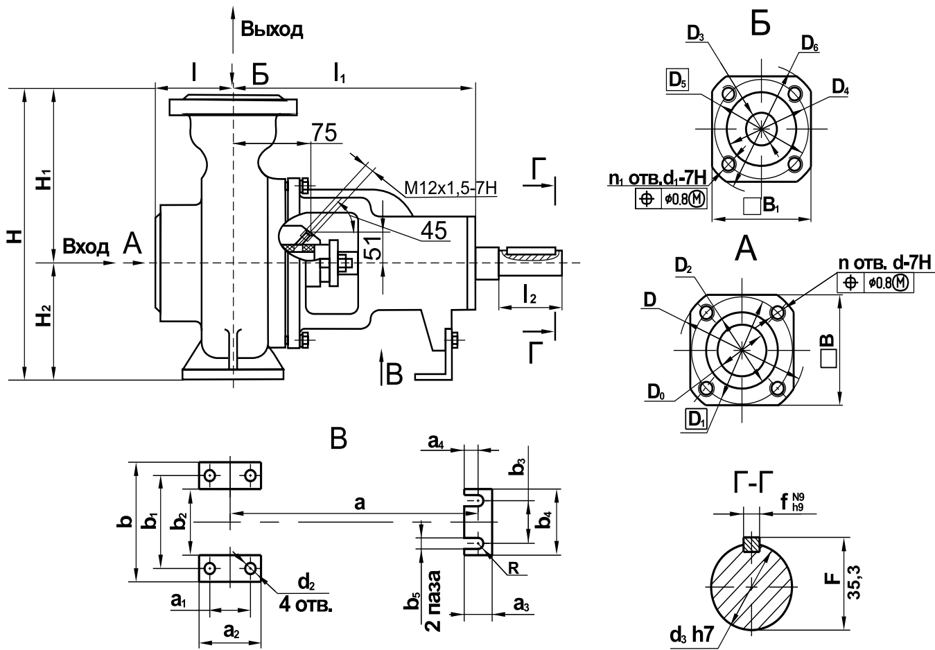
ГАБАРИТНЫЙ ЧЕРТЕЖ 2К80-65-160 И 2К100-80-160
