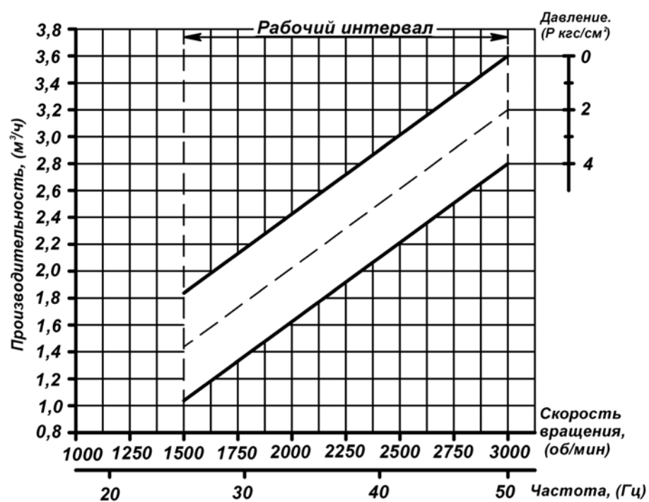
Электронасос Бурун СХ 3,6/4- Ч (ЧМ) 0,75/2
